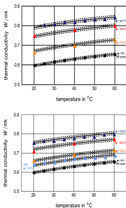
شکل ۵: رسانایی حرارتی بر حسب دما به ترتیب برای نانوسیال تیتانیا-آب و آلومینا-آب [۲۹].
