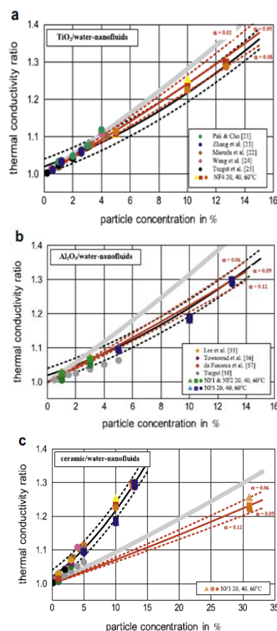
شکل ۴: نسبت رسانایی حرارتی بر حسب کسر حجمی ذرات برای نانوسیال (a) تیتانیا-آب، (b) آلومینا-آب و (c) اکسید سیلیسیم-آب [۲۹].
