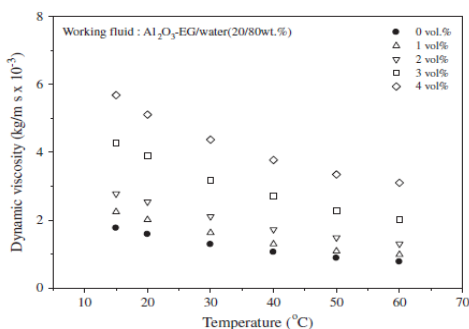
شکل ۸: مقایسه ویسکوزیته دینامیکی نانوسیال \text{Al}_2\text{O}_3\text{-EG/water} بر حسب دما برای کسرهای حجمی مختلف [۳۳].
