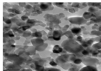
شکل ۶: تصویری از نانوذره \text{TiO}_2\text{-EG/water} [۳۳].
