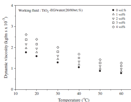
شکل ۷: مقایسه ویسکوزیته دینامیکی نانوسیال \text{TiO}_2\text{-EG/water} بر حسب دما برای کسرهای حجمی مختلف [۳۳].
