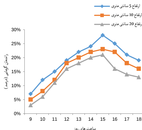
شکل ۱۲: نمودار مقایسه تغییرات راندمان گرمایی در سه ارتفاع ۵، ۱۰ و ۲۰ سانتی متری در ساعت های مختلف روز با جریان اجباری
