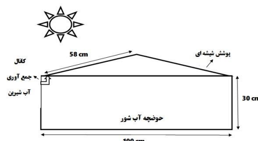
شکل ۸: نمای شماتیک دستگاه آب شیرین کن خورشیدی
