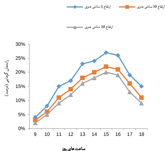
شکل ۱۱: نمودار مقایسه تغییرات راندمان گرمایی در سه ارتفاع ۵، ۱۰ و ۲۰ سانتی متری در ساعت های مختلف روز بدون جریان اجباری
