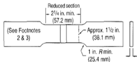
شکل ۲: نمونه آزمون کشش
