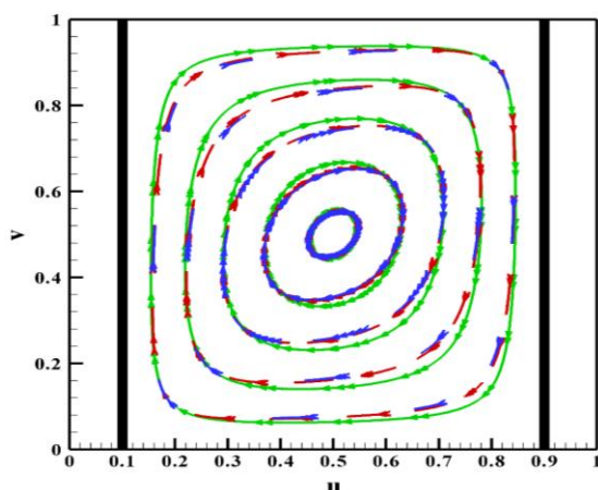
شکل (۶-ب): خطوط سبز رنگ (پیوسته) Ra=1 ، خطوط قرمز رنگ (خط چین) Ra=100 و خطوط آبی رنگ (خط چین با فاصله بیشتر نسبت به خط چین قرمز رنگ در Ra=100 ) در رابلی 10^5 .
