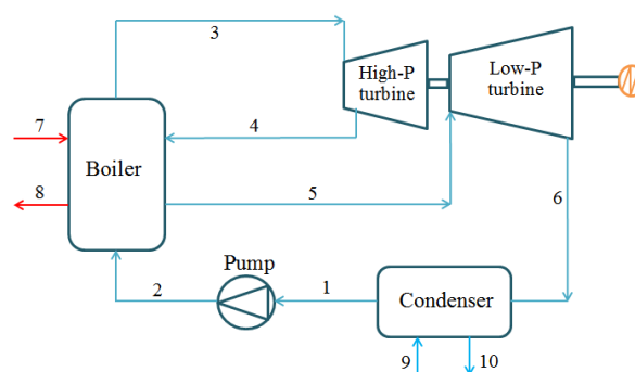
شکل ۲: شماتیک چرخه توربین بخار گرمایش مجدد
