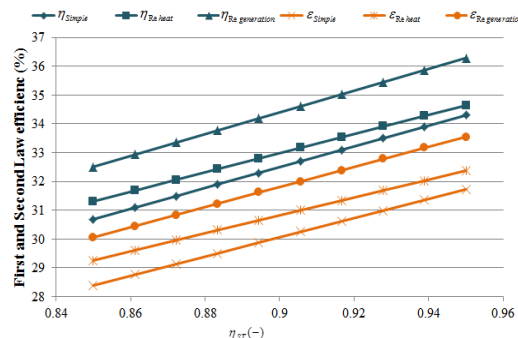
شکل ۱۳: تاثیر بازده آیزونتروپیکی توربین بخار بر روی بازده‌های قوانین اول و دوم ترمودینامیک در چرخه‌های توربین بخار ساده، توربین بخار گرمایش مجدد و توربین بخار بازیاب
