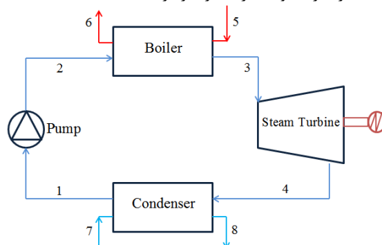
شکل ۱: شماتیک چرخه توربین بخار ساده
