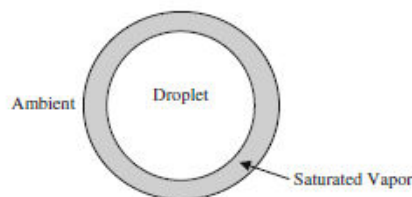
شکل (۳) مدل تبخیر قطره
