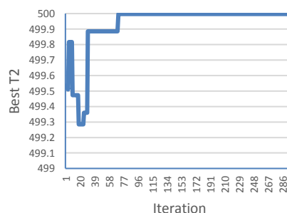
شکل ۵: روند بهینه شدن دمای خروجی از بویلر
