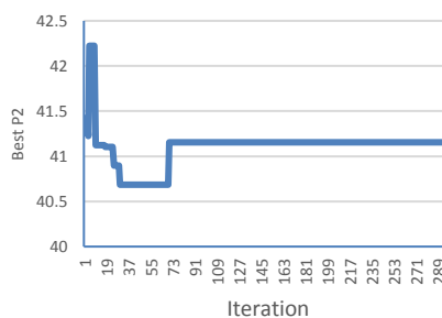
شکل ۶: روند بهینه شدن فشار خروجی از بویلر
