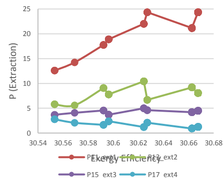
شکل ۹: تاثیر تغییرات فشارهای زیرکش توربین بر بازده اگزورژی
