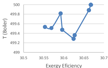
شکل ۷: روند تغییرات دمای خروجی از بویلر روی بازده انرژی
