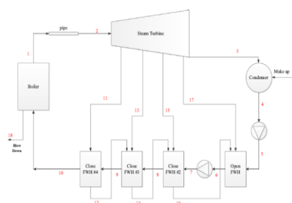
شکل ۱: فلو دیاگرام نیروگاه زرنده
