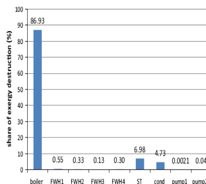
شکل ۲: مقایسه اتلاف انرژی در اجزاء مختلف نیروگاه
