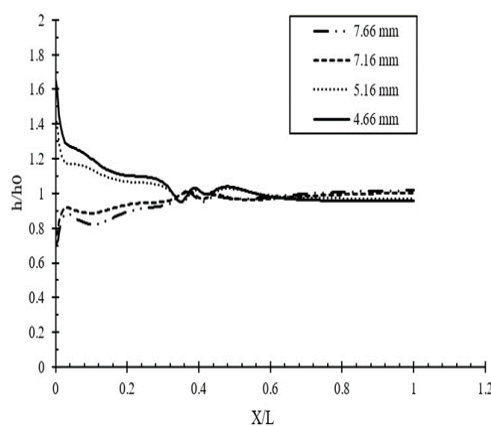
شکل ۵: تغییر قطر در رینولدز ثابت
