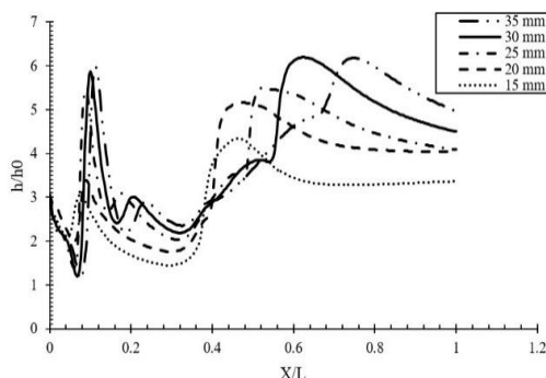
شکل ۱۰: برای پنج جته در فاصله‌های مختلف
