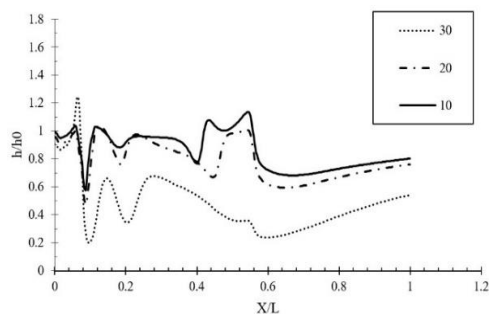
شکل ۱۶: مقایسه زاویه‌های مختلف تزریق با حالت صفر درجه برای پنج جت
