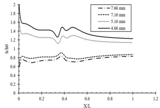
شکل ۶: تغییر قطر در دبی ثابت
