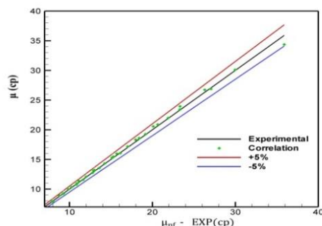
شکل ۱۰: مقایسه ویسکوزیته دینامیکی نتایج آزمایشگاهی کار حاضر با نتایج مدل
