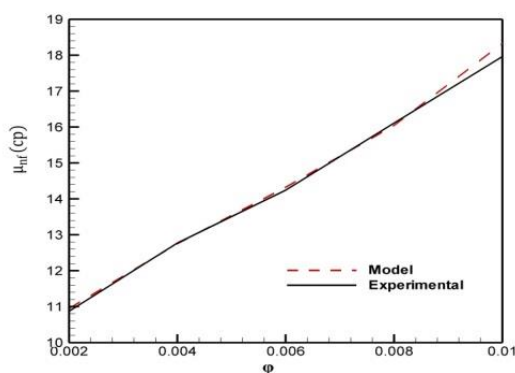
شکل ۹: نمودار مقایسه ویسکوزیته دینامیکی ارائه شده توسط مدل با نتایج آزمایشگاهی در کسر حجمی های مختلف
