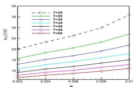
شکل ۶: تأثیر کسر حجمی بر ویسکوزیته دینامیکی نانوسیال اتیلن گلیکول-اکسیدروی در قطر ثابت ۲۰ نانومتر
