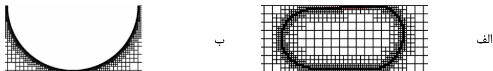
شکل ۲- گسسته سازی هندسه توسط روش AMR: (الف) با ۷ سطح پالایش انحنای (ب) با ۹ سطح پالایش برای مرز جامد منحنی.
