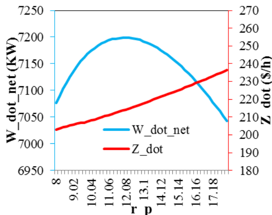
شکل ۱۵: تاثیر نسبت فشار کمپرسور بر کار کل و نرخ هزینه.
