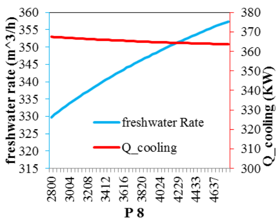
شکل ۱۱: تاثیر فشار ورودی به توربین بر دبی آب شیرین و سرمایه‌گذاری سیستم.
