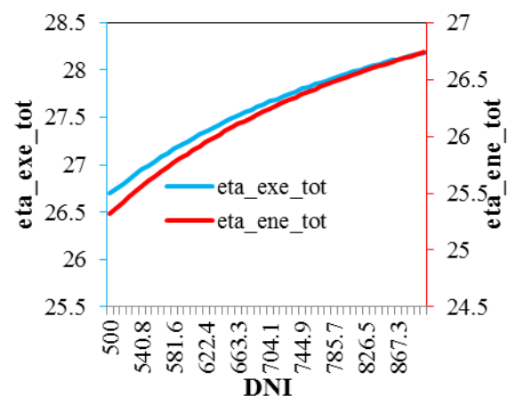
شکل ۳: تاثیر تابش خورشید بر بازده اگزرژی و بازده انرژی.
