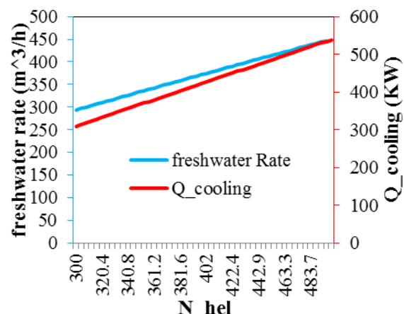
شکل ۱۰: تاثیر تعداد آینه‌ها بر دبی آب شیرین و سرمایش تولیدی سیستم.
