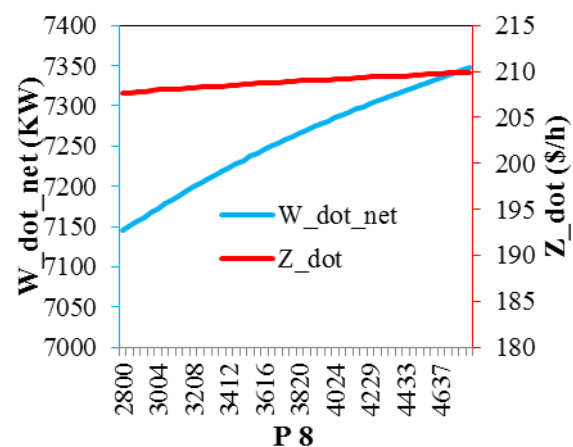
شکل ۱۲: تاثیر فشار ورودی به توربین بر کار کل و نرخ هزینه سیستم.
