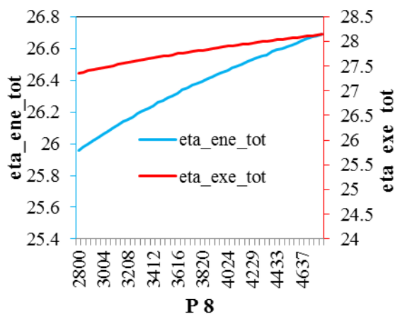
شکل ۱۱: تاثیر فشار ورودی به توربین بر بازده انرژی و بازده انرژی.
