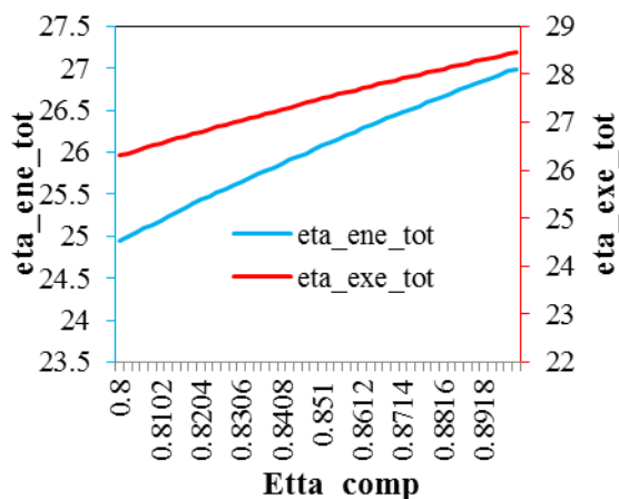
شکل ۵: تاثیر بازده کمپرسور بر بازده اگزرژی و بازده انرژی.
