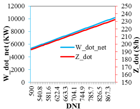
شکل ۳: تاثیر تابش خورشید بر کار کل و نرخ هزینه سیستم.
