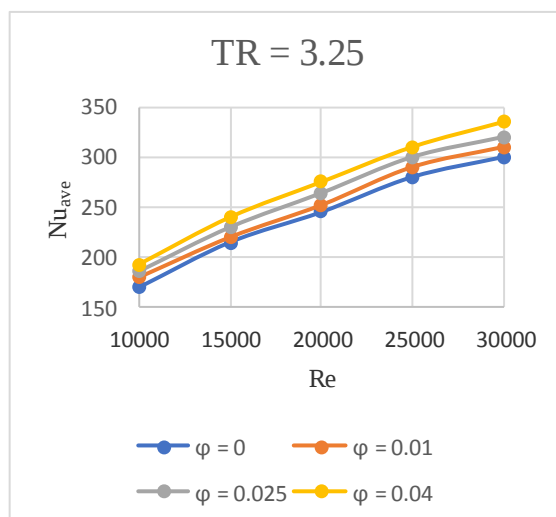
شکل ۹ مقایسه عدد ناسلت با افزایش عدد رینولدز در نسبت پیچ ۴ شکل ۱۰ مقایسه عدد ناسلت با افزایش عدد رینولدز در نسبت پیچ ۳/۲۵ برای درصد های مختلف حجمی نانو ذرات
