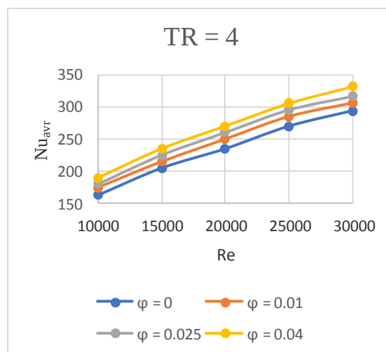
شکل ۹ مقایسه عدد ناسلت با افزایش عدد رینولدز در نسبت پیچ ۴ شکل ۱۰ مقایسه عدد ناسلت با افزایش عدد رینولدز در نسبت پیچ ۳/۲۵ برای درصد های مختلف حجمی نانو ذرات
