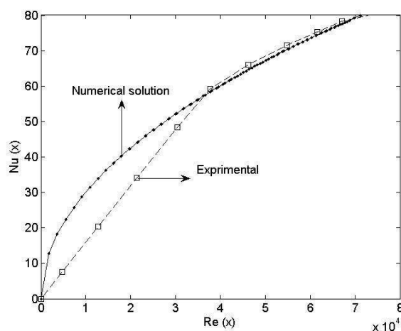
شکل ۹- نمودار تغییرات Nu(x) به Re(x) مقایسه‌ی Numerical solution به Experimental با Re=1.72 \times 10^5 Pr=0.71 و Nu=122.54
