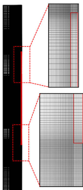
شکل ۵- مش‌بندی ناحیه محاسباتی صفحه فلزی ایستاده
