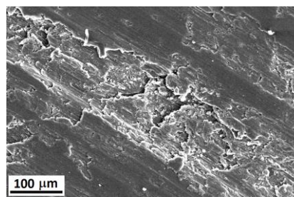
شکل(۲): سطح سایش یافته کامپوزیت Al-15SiO 2
