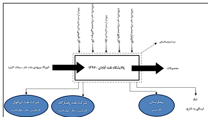
شکل ۲: ترسیم حجم کنترل محاسباتی و جریان های مواد و انرژی
