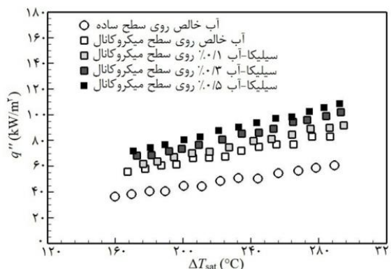
شکل ۲۳- منحنی جوشش فیلمی نانوسیال سیلیکا-آب روی سطح میکروکانال
