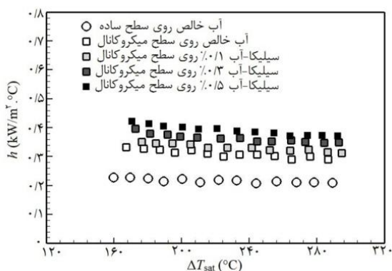
شکل ۲۲- منحنی ضریب انتقال حرارت جوشش فیلمی بر حسب اختلاف دمای مازاد برای نانوسیال سیلیکا-آب روی سطح میکروکانال
