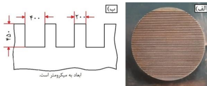
شکل ۵- تصویر و شماتیک سطح میکروکانال مورد استفاده در تحقیق حاضر
