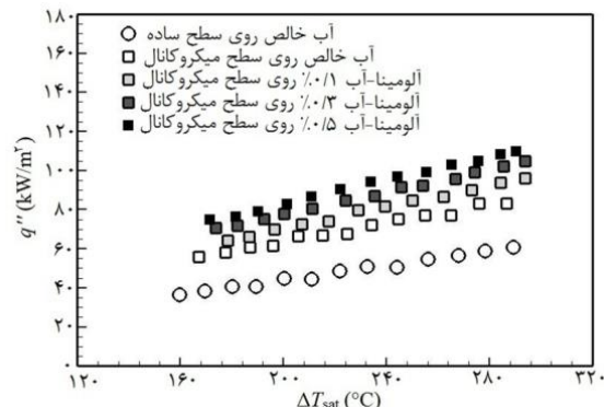
شکل ۲۱- منحنی جوشش فیلمی نانوسیال آلومینا-آب و آب خالص روی سطح میکروکانال
