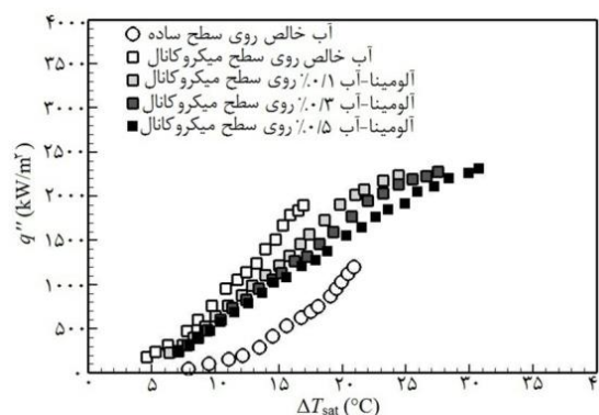
شکل ۱۳- منحنی جوشش هسته‌ای نانوسیال آلومینا-آب و آب خالص روی سطح میکروکانال
