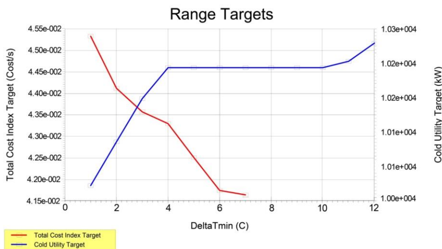
شکل ۶: نمودار هدف گذاری برای میزان مصرف بار خارجی سرد و هزینه‌های سرمایه بر اساس \Delta T_{min} متفاوت (محل تقاطع نقطه بهینه مصرف انرژی معادل ۲/۳ درجه سانتی‌گراد)
