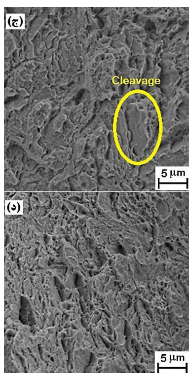
شکل (۵): سطح شکست (الف) نمونه خام (ب) نمونه کوئنچ شده (ج) نمونه یک مرحله بازپخت شده و (د) نمونه دو مرحله بازپخت شده.
