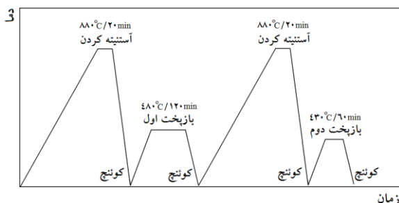
شکل(۲): سیکل کلی عملیات حرارتی انجام شده در تحقیق.
