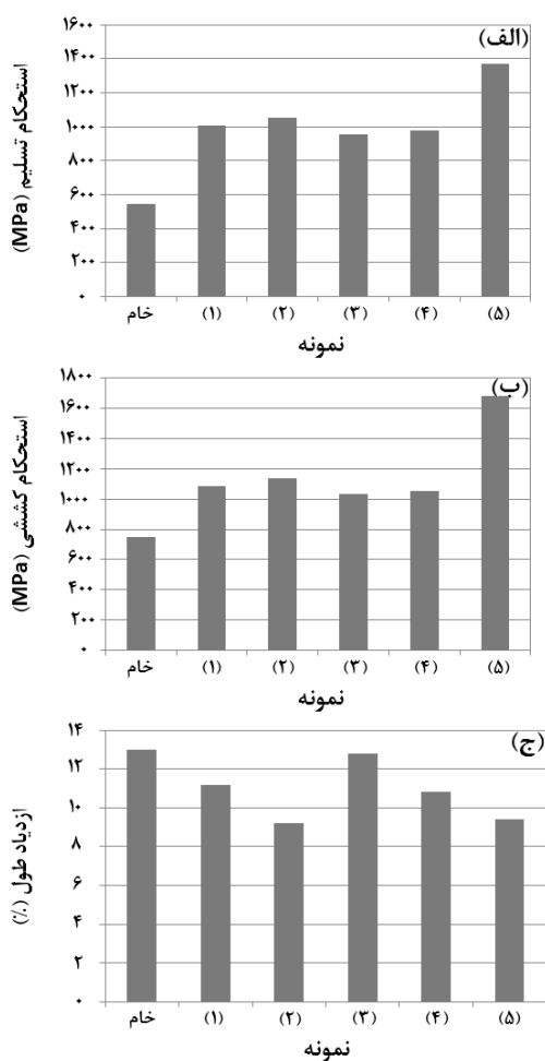
شکل (۴): نمودار تغییرات (الف) استحکام تسلیم (ب) استحکام کششی و (ج) ازدیاد طول در نمونه های عملیات حرارتی شده تحت شرایط مختلف.
