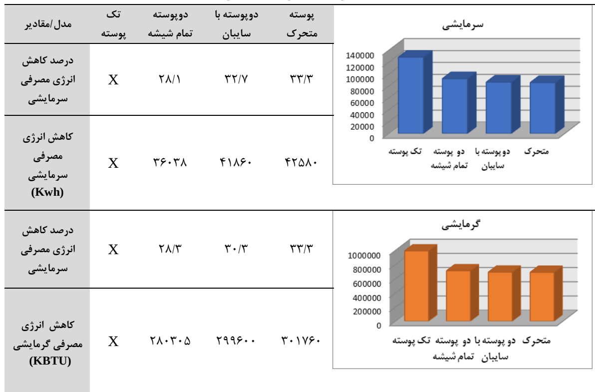
جدول ۲- نمودار مقایسه‌ای میزان انرژی مصرفی (گرمایشی و سرمایشی) و تغییرات آن بین مدل‌های مورد مطالعه
