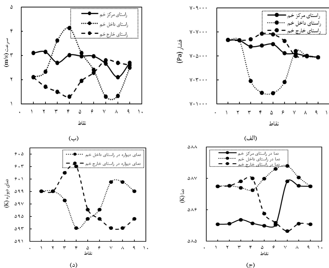
شکل ۸: نمودار روند تغییر پارامترها در راستای مرکز، داخل و خارج خم (الف) فشار سیال (ب) سرعت سیال (ج) دمای سیال (د) دمای دیواره خارجی کوئل
