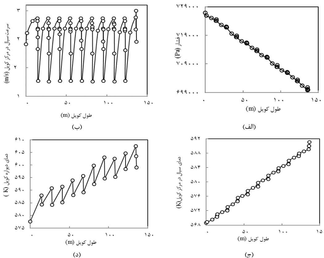
شکل ۶: نمودار روند تغییر پارامترها در راستای مرکز در طول کویل (الف) فشار سیال (ب) سرعت سیال (ج) دمای دیواره (د) دمای سیال خارجی کویل
