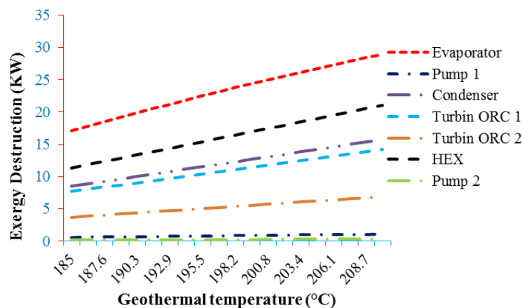
شکل ۶- بررسی تاثیر تغییرات دمای زمین‌گرمایی (T1) بر میزان تخریب اگزورژی اجزاء سیستم
