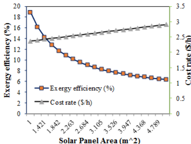
شکل ۹: بررسی تاثیر تغییرات مساحت پنل خورشیدی (Solar Panel) بر روی خروجی های سیستم
