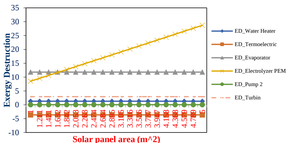
شکل ۱۳: بررسی تاثیر تغییرات مساحت پنل خورشیدی ( A_{\text{Solar Panel}} ) بر میزان تخریب اگزورژی اجزا سیستم
