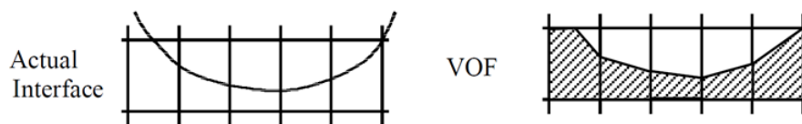
شکل ۳- محل تماس دو فاز در حالت واقعی (بالا) و با روش اویلری حجم مایع (پایین)
