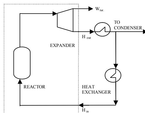
شکل ۳- مدلسازی توربین انبساطی و راکتور
