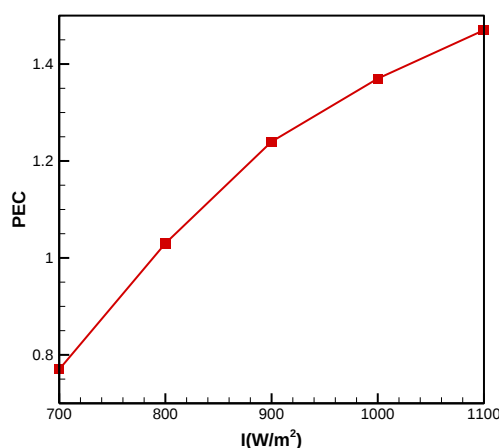
شکل ۴- الف. مقدار عدد ناسلت متوسط، ب. افت فشار، ج. ضریب کارایی، برای مقادیر مختلف شدت تابش خورشیدی و عدد رینولدز ۳۰۰۰ در کانال ساده
