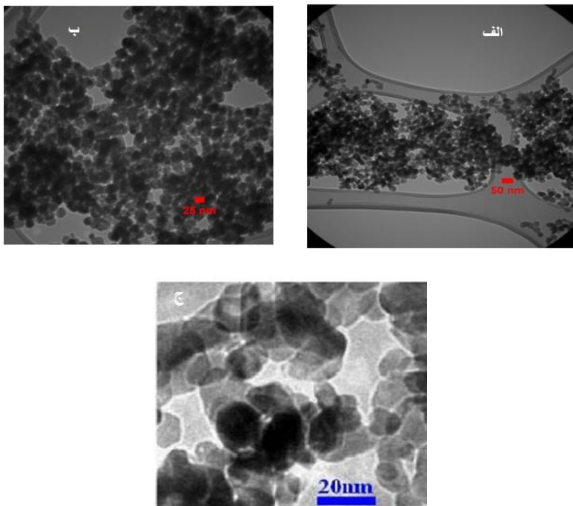
شکل ۱ - عکس TEM نانوذرات استفاده شده (الف) اکسید آلومینیوم (ب) اکسید منیزیم (ج) اکسید روی
