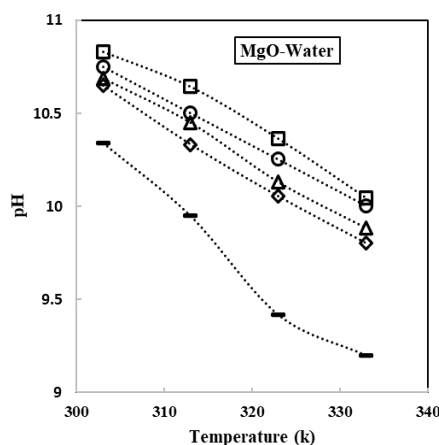
شکل ۵. مقایسه pH نانوسیال MgO به صورت تابعی از دما در غلظت‌های مختلف
