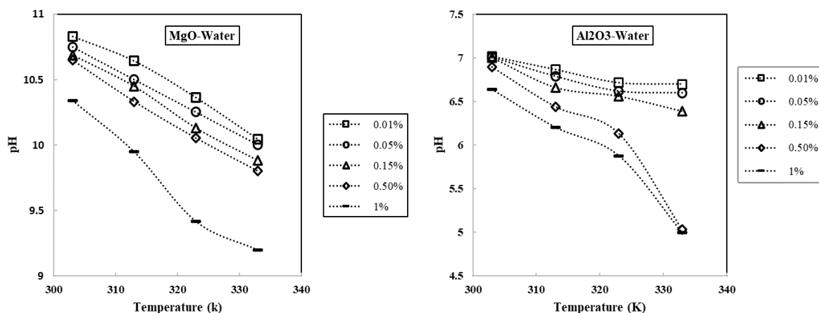
شکل ۴. مقایسه pH نانوسیال Al_2O_3 به صورت تابعی از دما در غلظت‌های مختلف
