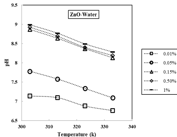
شکل ۸. مقایسه pH نانوسیال ZnO به صورت تابعی از دما در غلظت های مختلف
