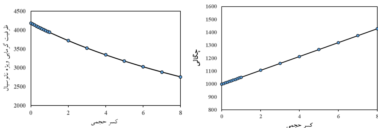
شکل ۴- نمودار تغییرات ظرفیت گرمایی ویژه نانوسیال نسبت به کسر حجمی نانوسیال.
