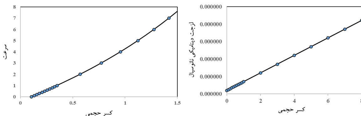
شکل ۶- نمودار سرعت در کسر حجمی مختلف.
