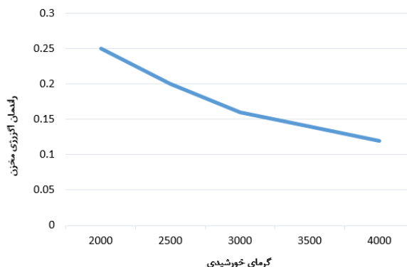
شکل (۳): راندمان انرژی مخزن نسبت به گرمای خورشیدی
