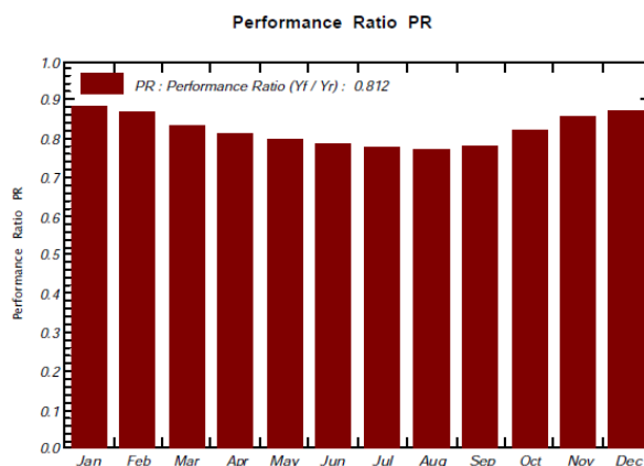
شکل ۱۰: ضریب عملکرد نیروگاه در ماه‌های مختلف سال (نرم افزار PVSyst)
