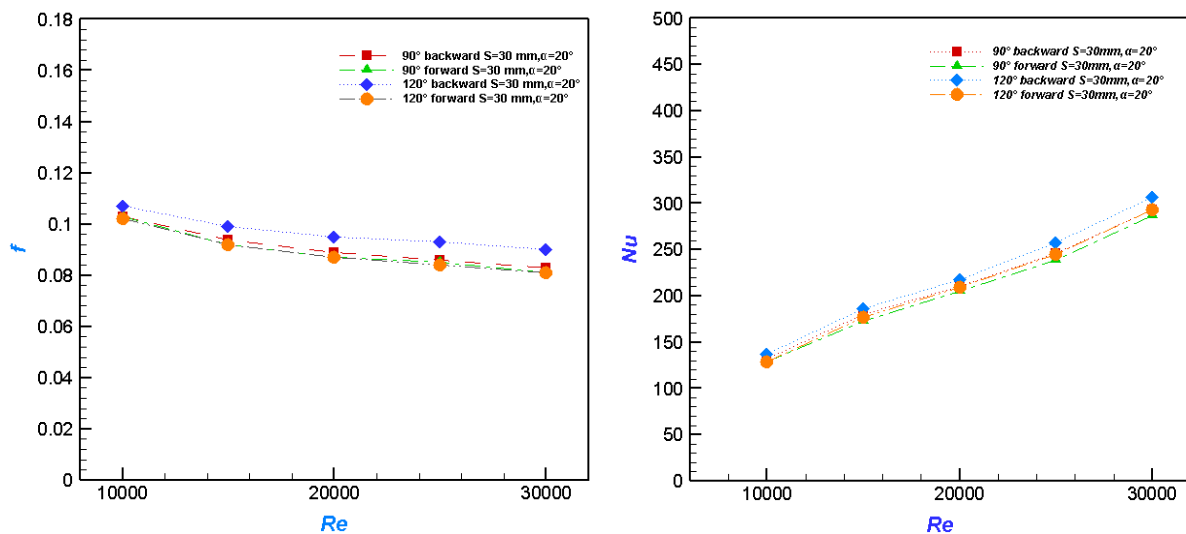
شکل (۹): نمودار تاثیر عدد رینولدز بر ضریب اصطکاک
