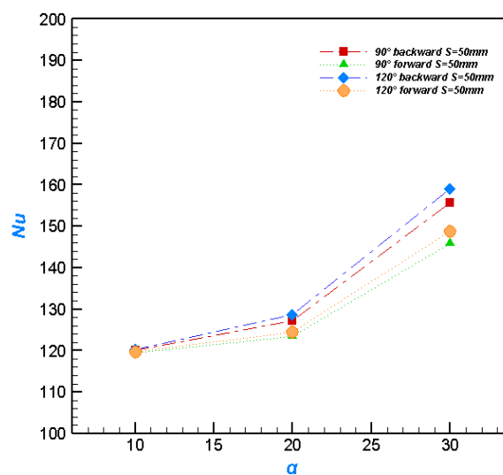
شکل (۱۴): نمودار تاثیر زاویه آشفته‌ساز بر عدد ناسلت
