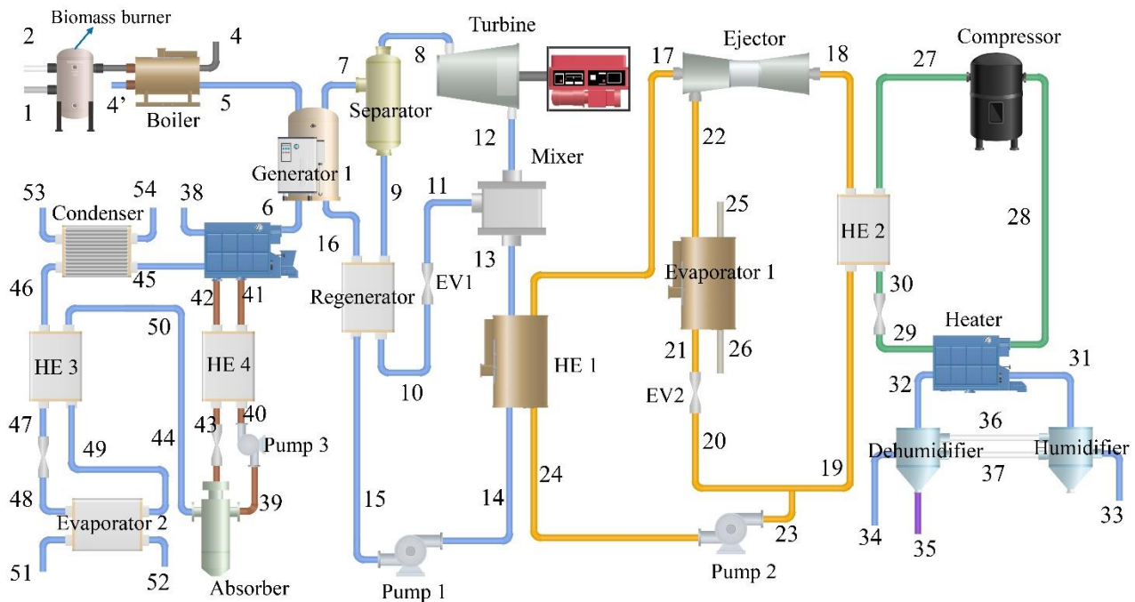
شکل ۱ - نمای شماتیک سیستم پیشنهادی
