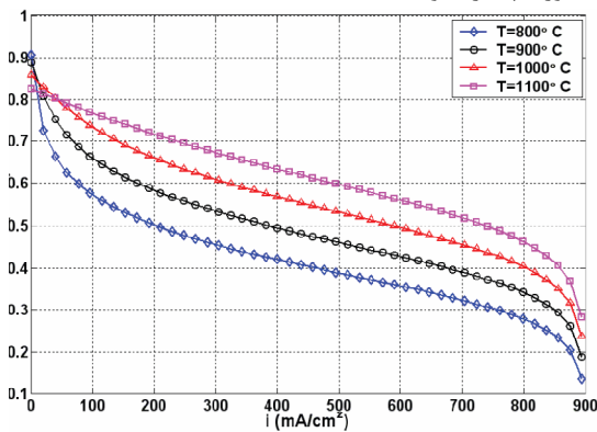
شکل ۳- نمودار ولتاژ-چگالی جریان پیل سوختی اکسید جامد لوله‌ای در دماهای مختلف و فشار ۱ bar [۱۰]
