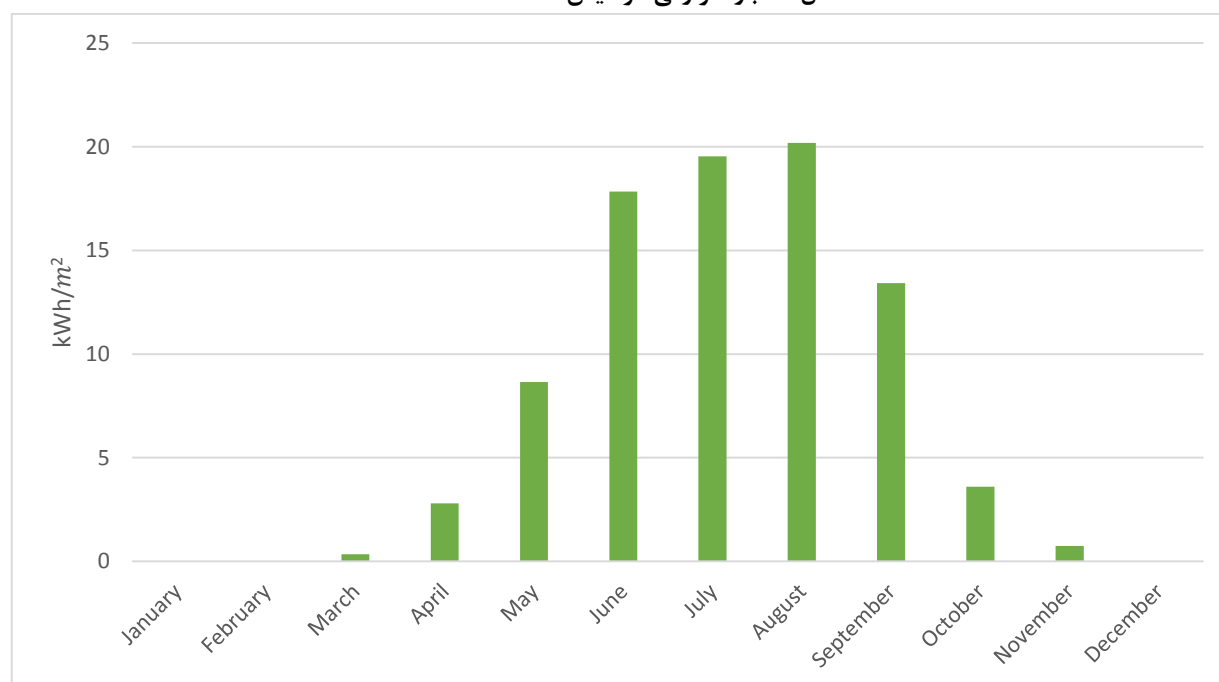
شکل ۵- بار حرارتی سرمایش فضا \text{kWh/m}^2
