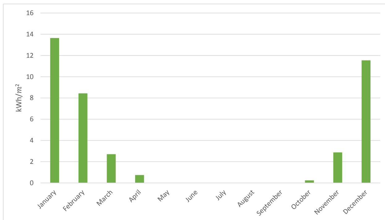
شکل ۴- بار حرارتی گرمایش فضا \text{kWh/m}^2
