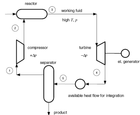
شکل ۳- نحوه یکپارچه سازی توربین گاز با راکتور شیمیایی [۵۰]
