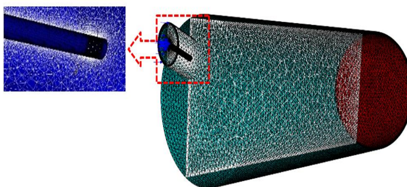
شکل ۵: شبکه تولید شده برای کوره
