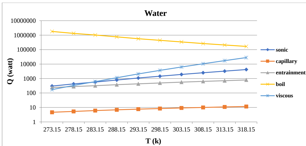
شکل ۴- نتیجه محاسبات با استفاده از ۱۰۰ مش بر اینچ وایر صفحه‌ای در ساختار فتیله سه لایه جهت آب.
