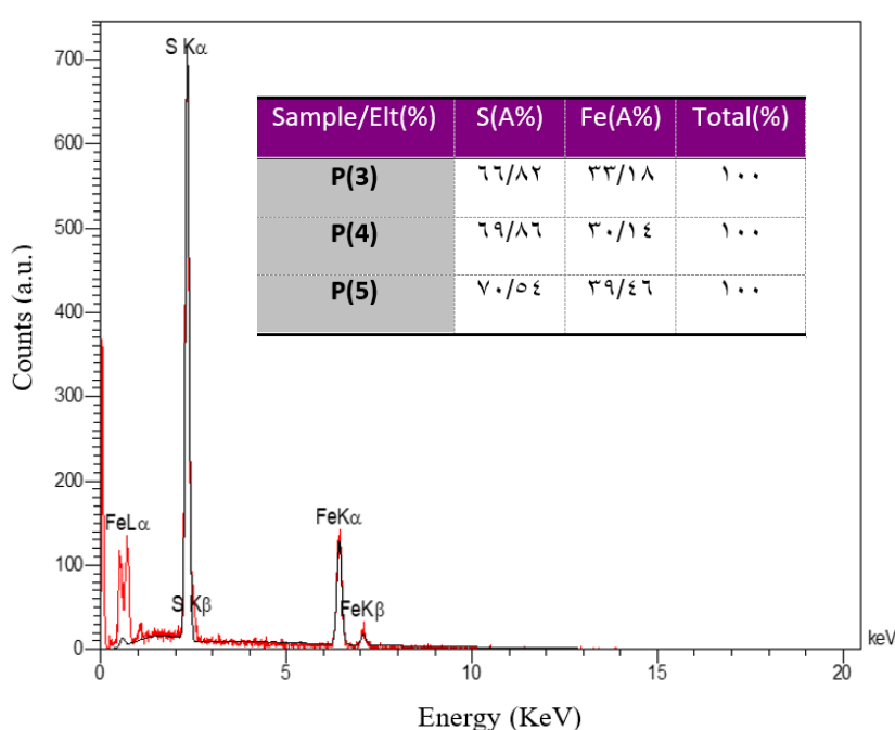
شکل (۴): نتایج EDX نمونه‌های P(3)، P(4) و P(5)
