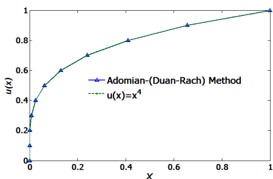
شکل ۲: مقایسه حل روش اصلاحی آدومین-دوان راج با جواب دقیق مسئله
