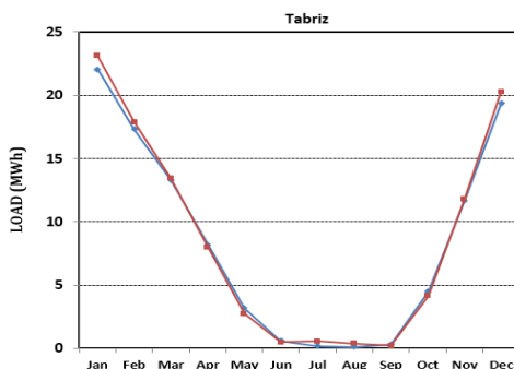
شکل (۱۰): بار حرارتی سقف سبز در دو حالت پایه و ثانویه برای ساختمان مورد مطالعه واقع در شهر تبریز
