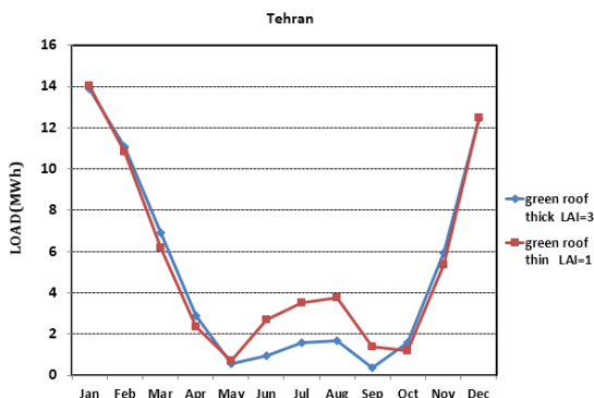
شکل (۹): بار حرارتی سقف سبز در دو حالت پایه و ثانویه برای ساختمان مورد مطالعه واقع در شهر تهران
