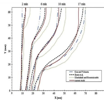
شکل (۲-۲): موقعیت های کسر ذوب در زمان های مختلف [۵،۴،۶]
