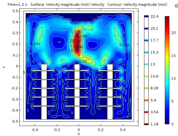
شکل (۹-۴): کانتور سرعت برای سه هیت پایپ با نانو سیال
