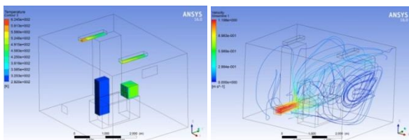
شکل (۹): حرکت جریان هوا و کانتور دما برای نمونه شماره ۷
