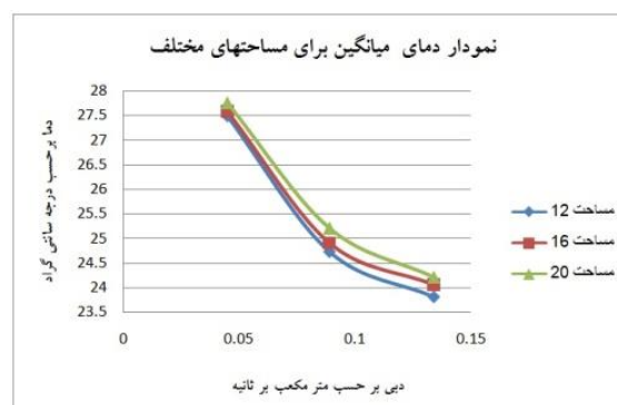
شکل (۲۷): دمای میانگین اتاق برای مساحت های مختلف بر حسب دبی های مختلف
