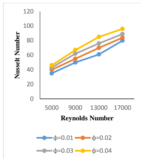
شکل ۴: عدد ناسلت در درصدهای حجمی مختلف نانوذره
