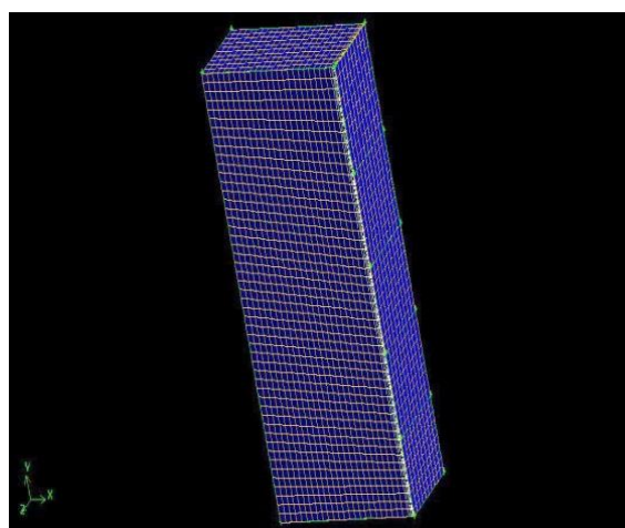
شکل ۲- شبکه‌بندی شکل صفحه فلزی به ابعاد 1m×0.2m×0.005m
