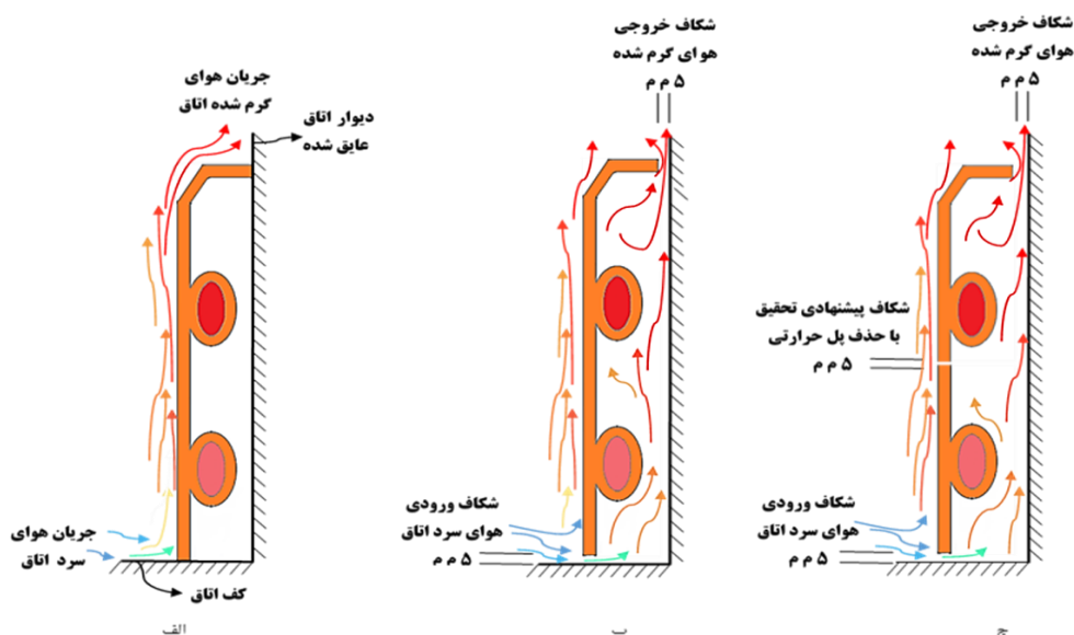
شکل ۲- تغییرات ساختاری پروفیل های گرمایشی قرنیزی. (الف) مورد متداول (مورد ۱)، (ب) مورد اصلاح شده مطالعه قبلی (مورد ۲) [۱]، (ج) مورد مطالعه حاضر (مورد ۳)
