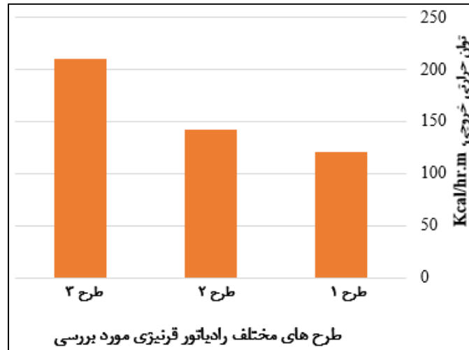
شکل ۶. نمودار مقایسه برآورد توان گرمایشی رادیاتور های قرنیزی نوع ۱ و ۲ و ۳ مطابق گزارش آزمایشگاه استاندارد
