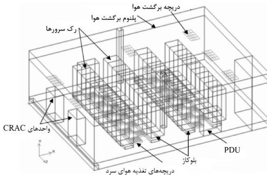
شکل ۱: شکل شماتیک مرکز داده مورد مطالعه
