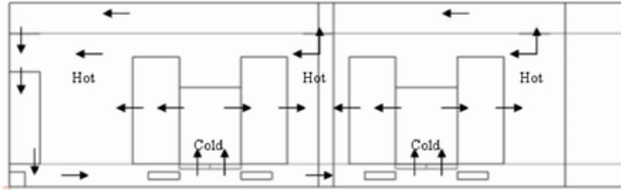
شکل ۲: چیدمان راهرو سرد و گرم و مسیر جریان هوا در داخل سالن مرکز داده
