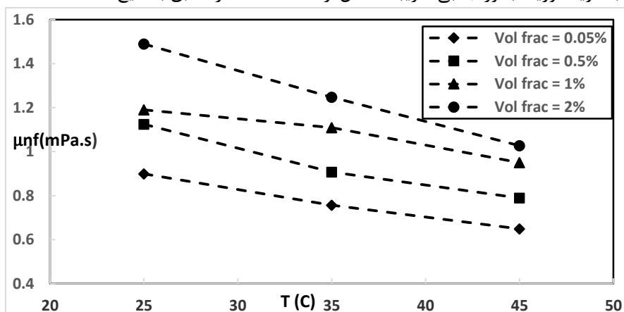
شکل ۱۱. تاثیر دما بر ویسکوزیته نانوسیال اکسید آلومینیم-آب
