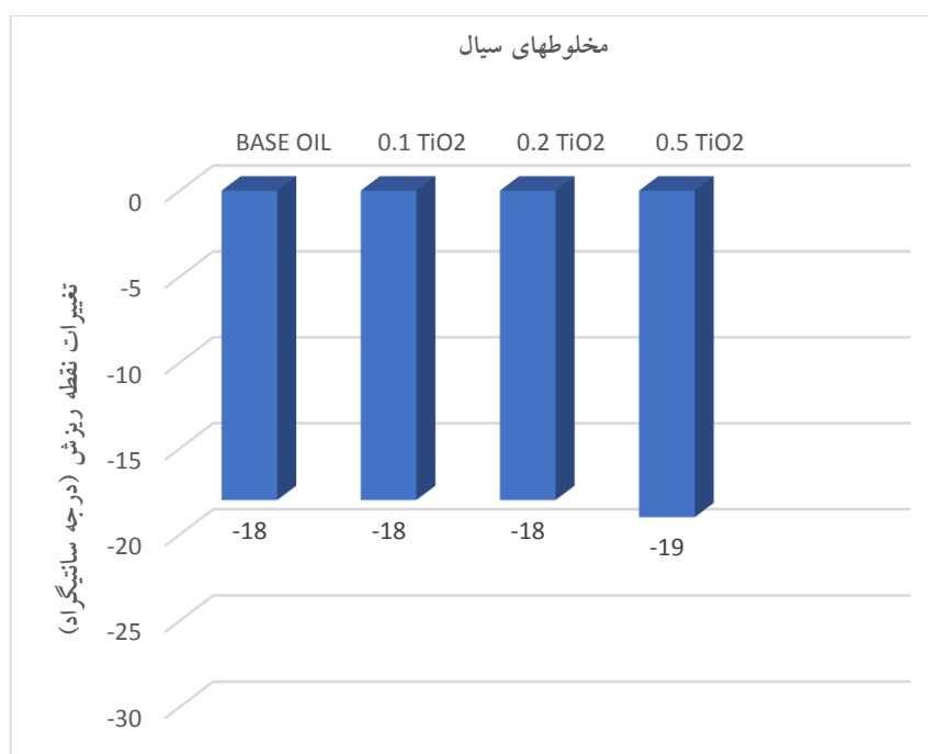
شکل ۱۵- تغییرات نقطه‌ی ریزش نمونه‌ها.
